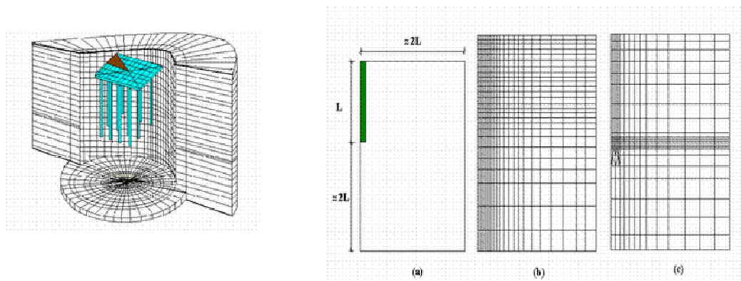
Figura 1. Modelación de la Cimentación. Modelo axial-simétrico.
